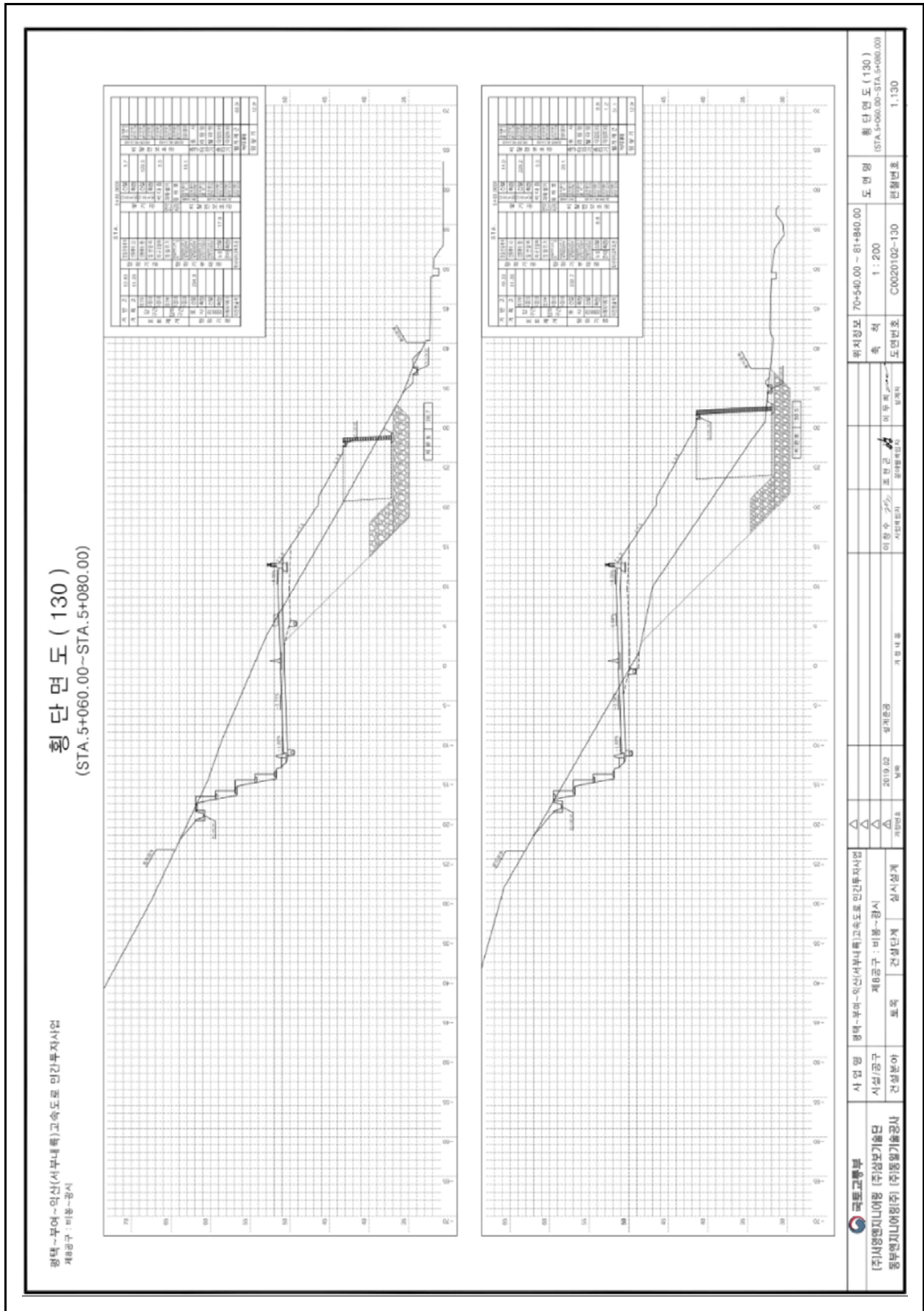
【그림 4.18.3】 횡단면도1
